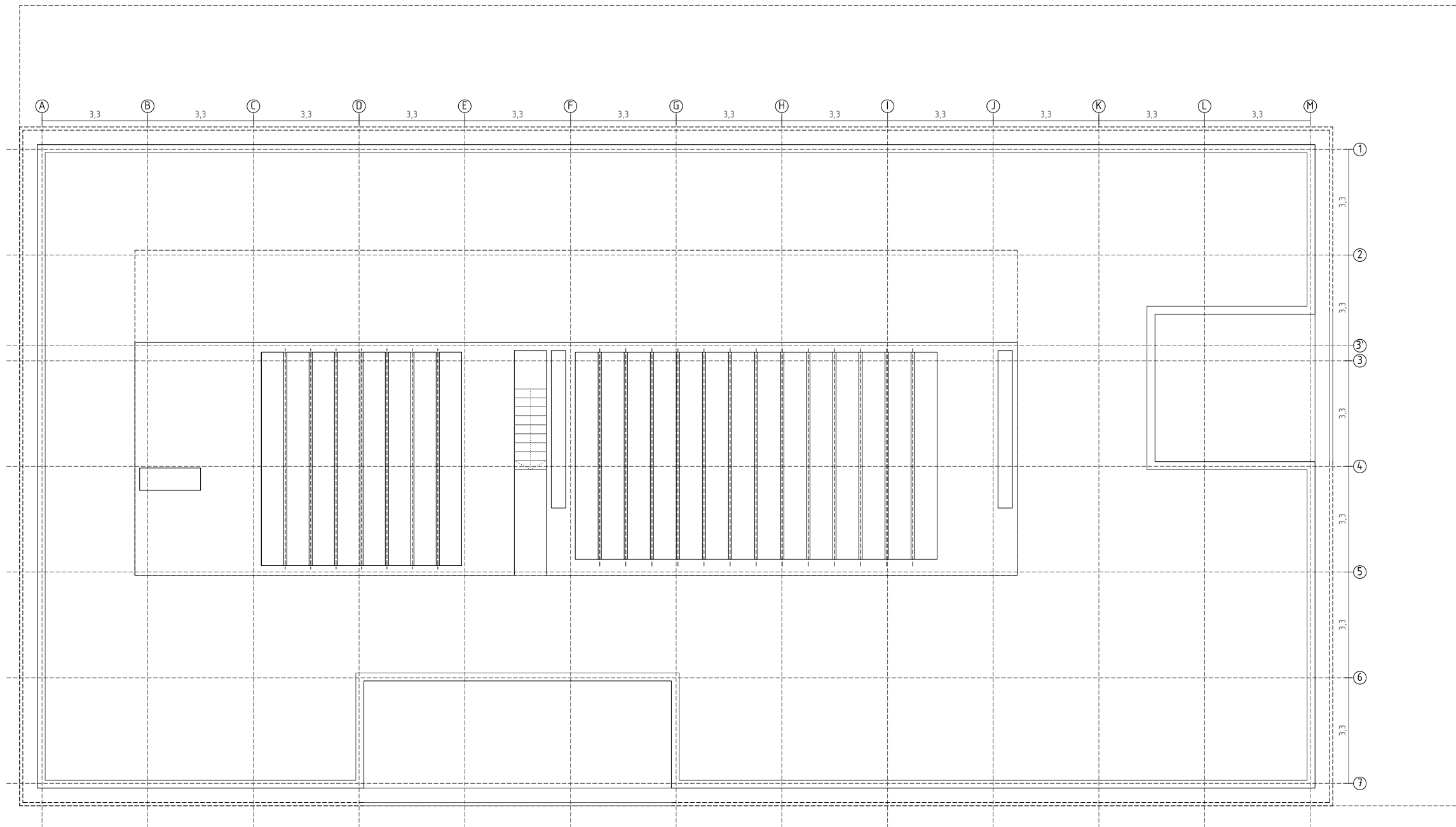
E 1:150 PLANTA DE CUBIERTAS
