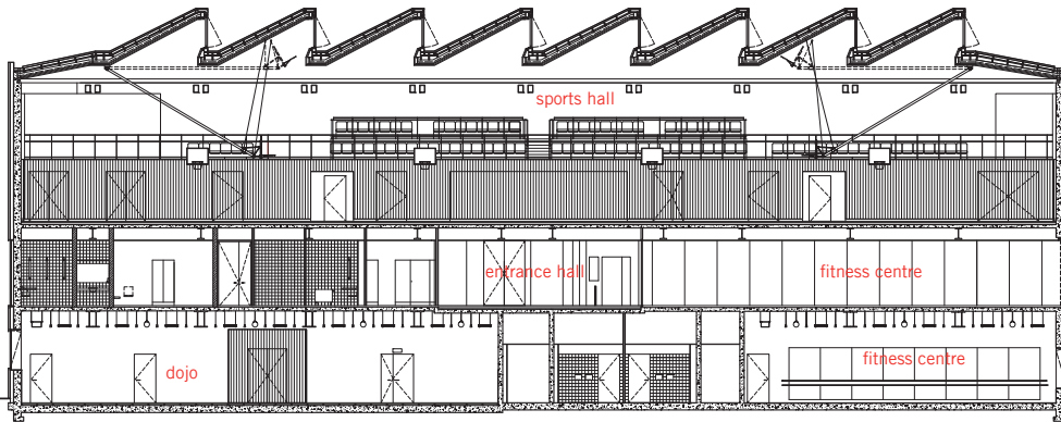
Longitudinal section
