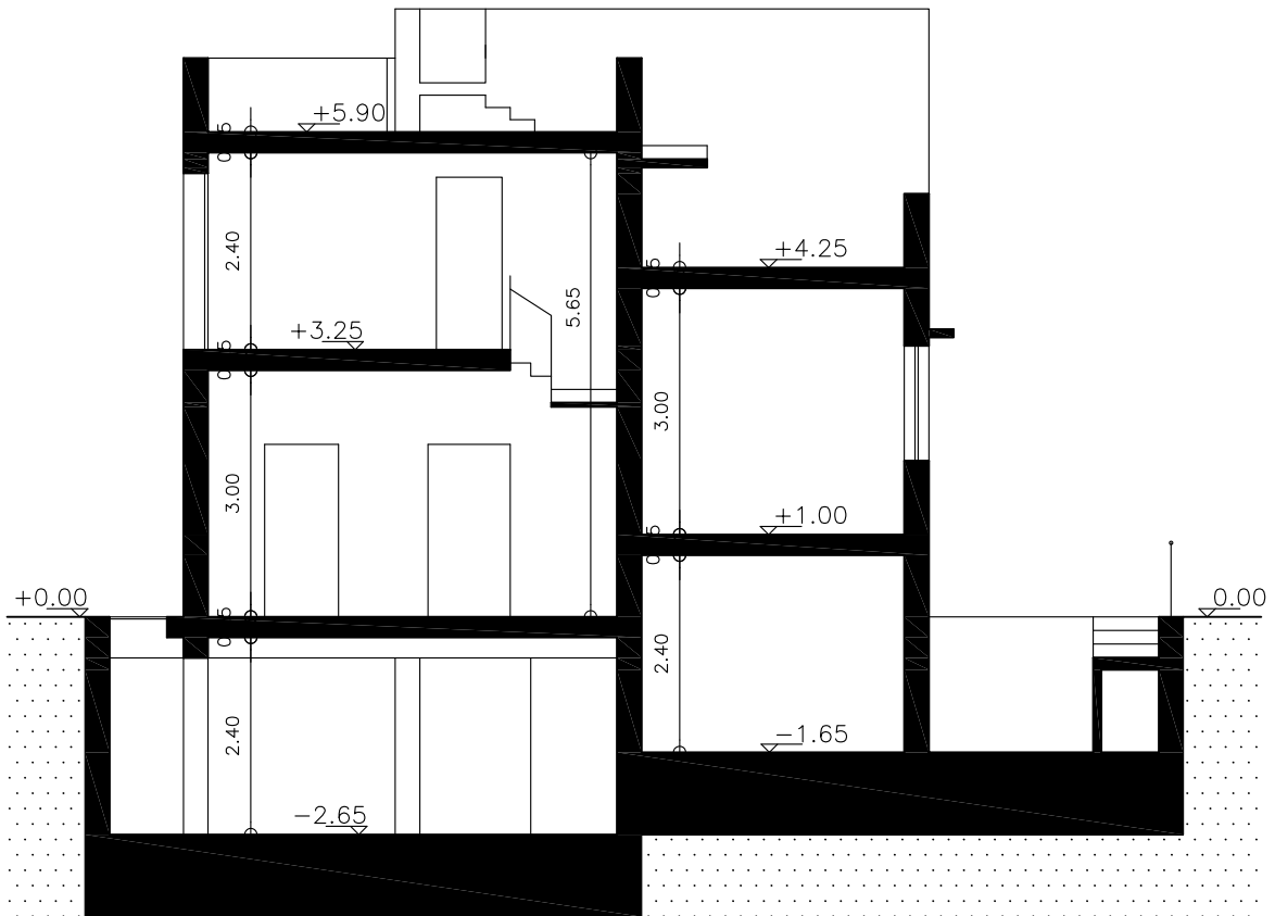
sezione B-B'
