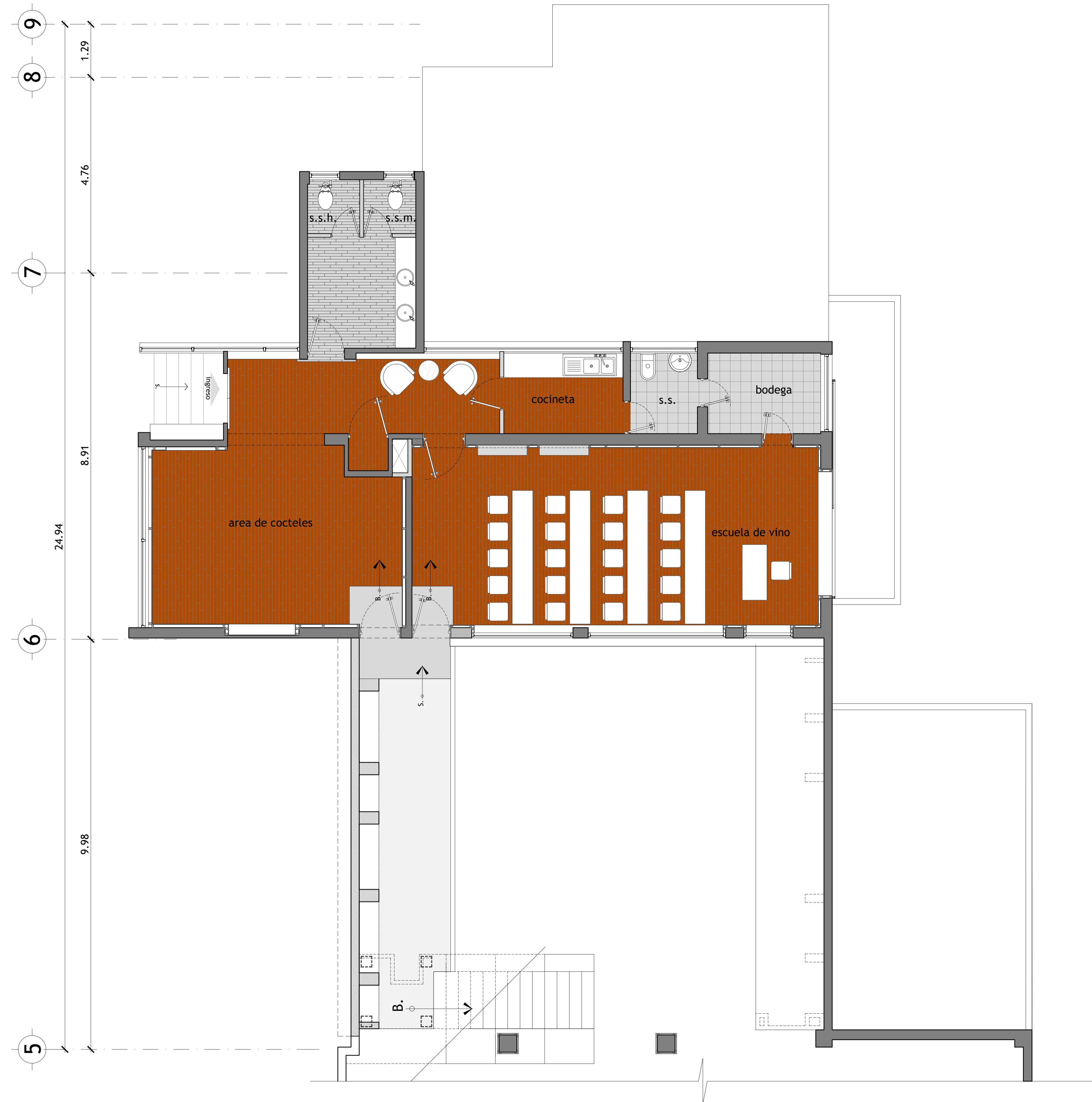
planta arquitectónica escala 1/50
