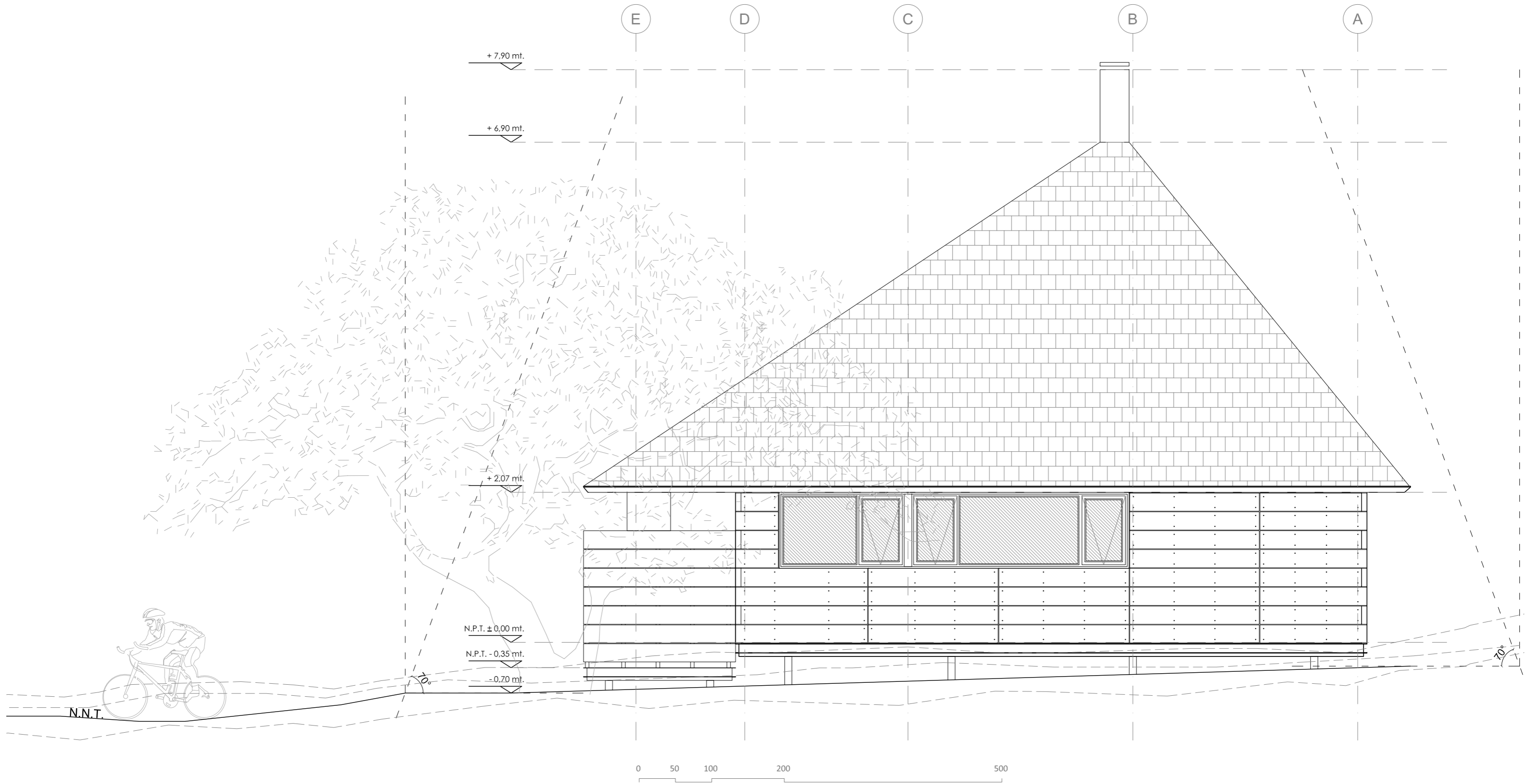
elevación oriente
