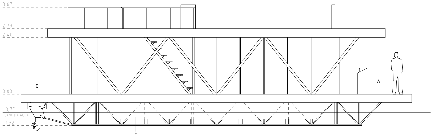
PERFIL A
