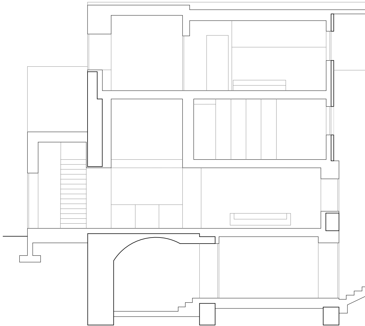
coupe longitudinale
