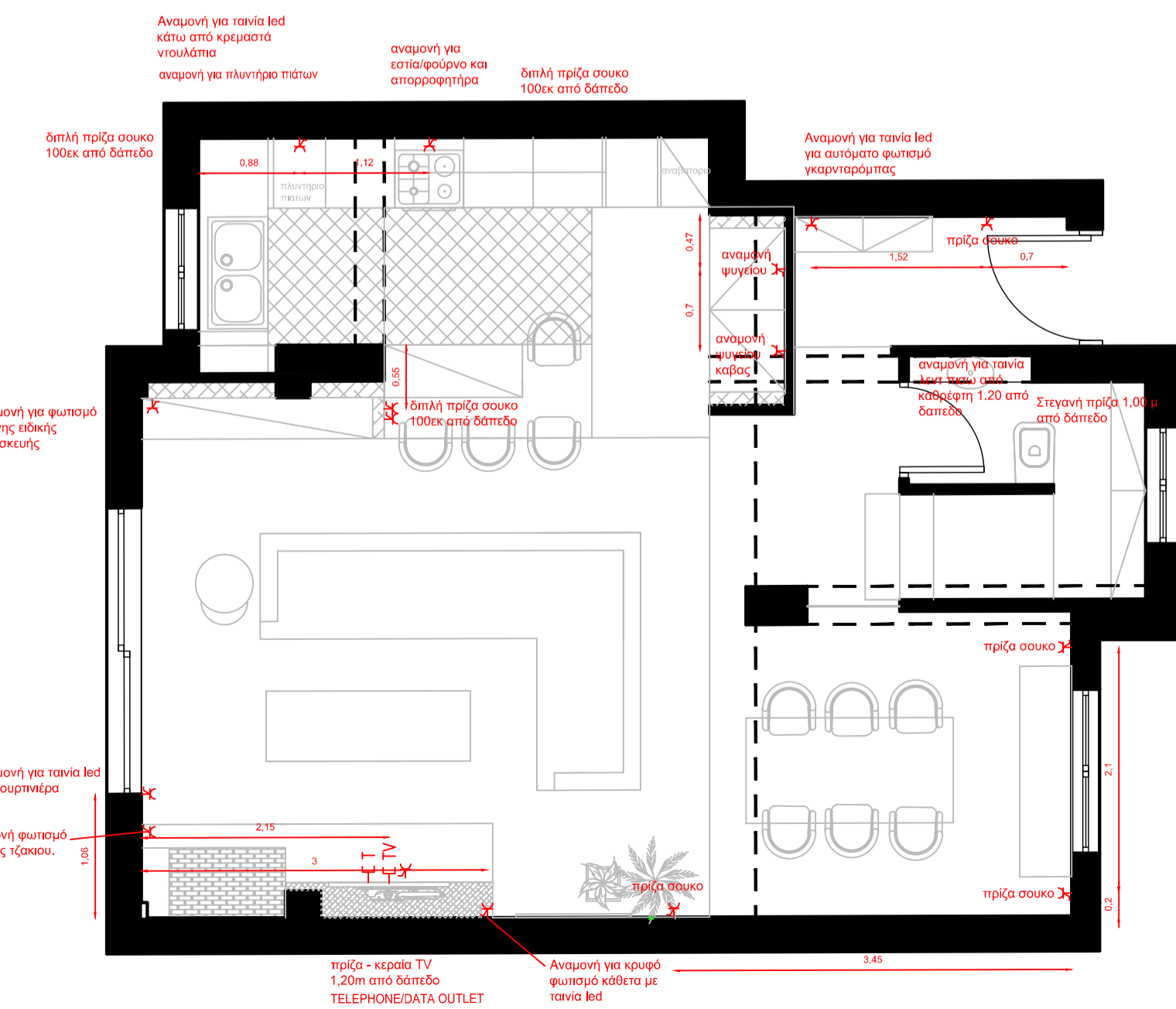
ΗΛΕΚΤΡΟΛΟΓΙΚΟ ΣΧΕΔΙΟ
