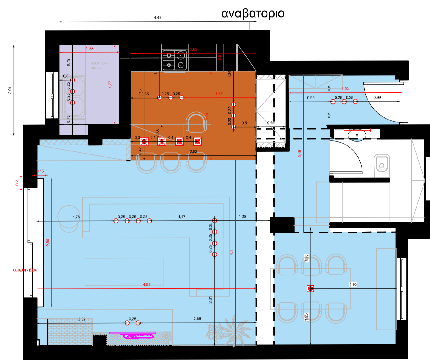
ΑΝΟΨΗ ΙΣΟΓΕΙΟ
