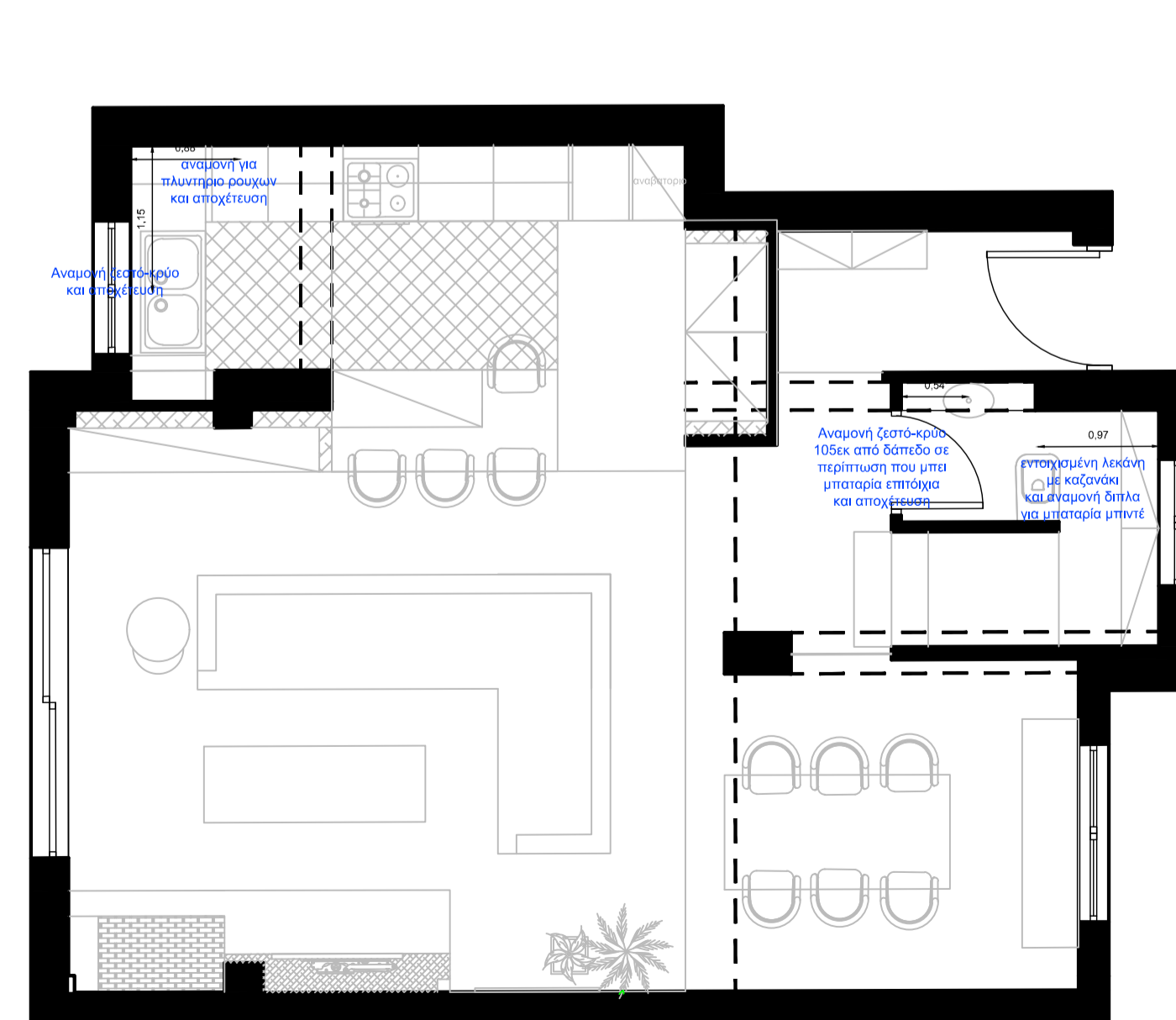
ΥΔΡΑΥΛΙΚΟ ΣΧΕΔΙΟ
