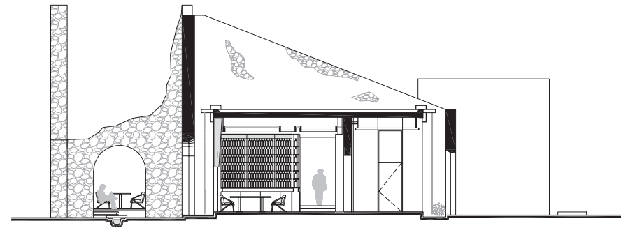
SECCIÓN B-B' SECTION B-B'
