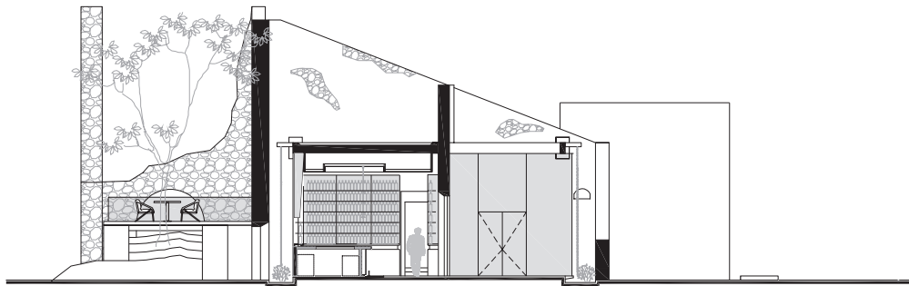
SECCIÓN A-A' SECTION A-A'
