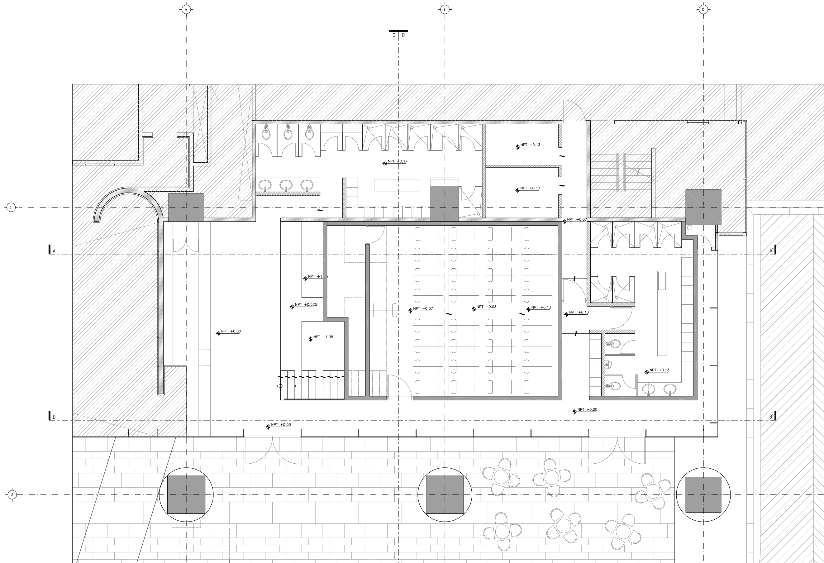
1 PLANTA BAJA SICLO
