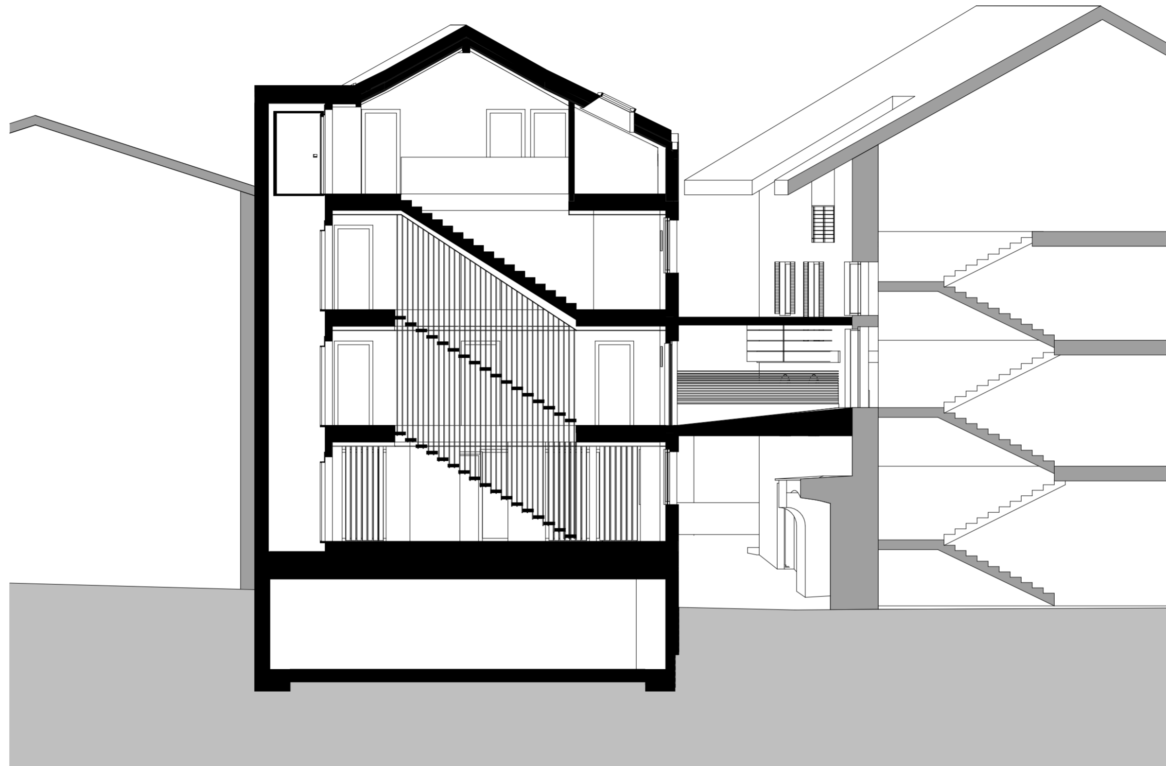
Section A-A S 1:100
