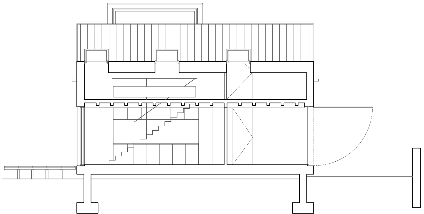
Corte C
