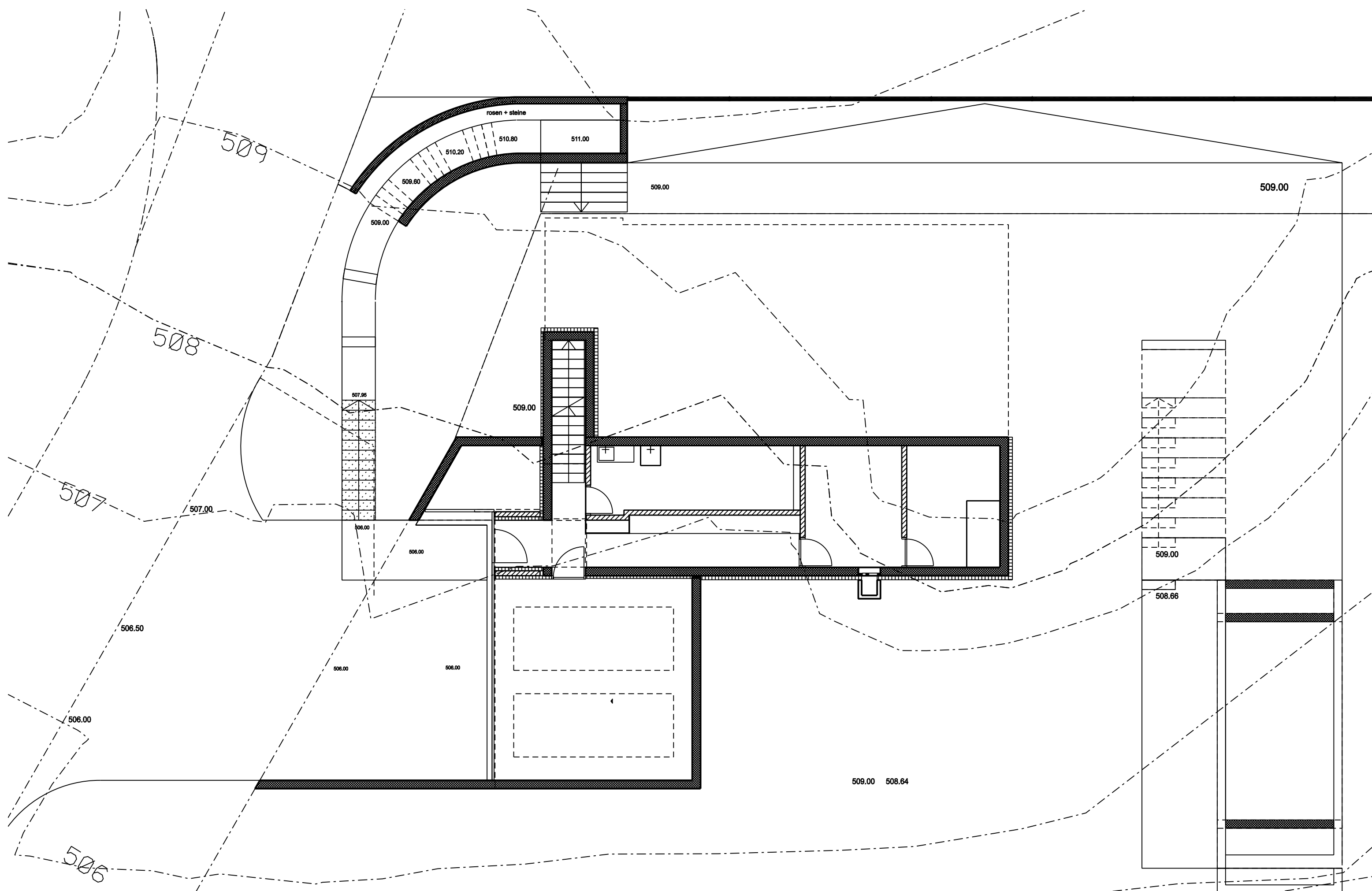
feldbalz house 1:100 basement gus wüstemann ma eth sia coac
