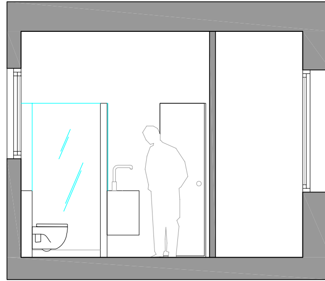
Sección CC'
