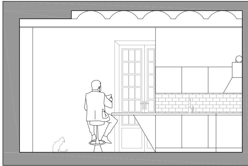
Sección AA'
