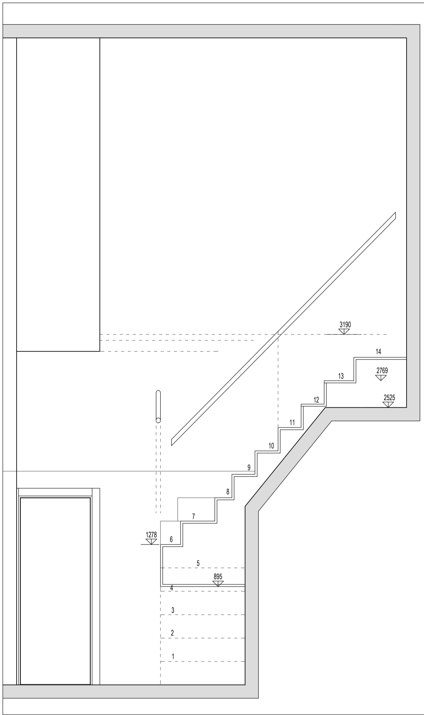
DISEGNI ESECUTIVI SCALA TORRETTA scala 1:25
