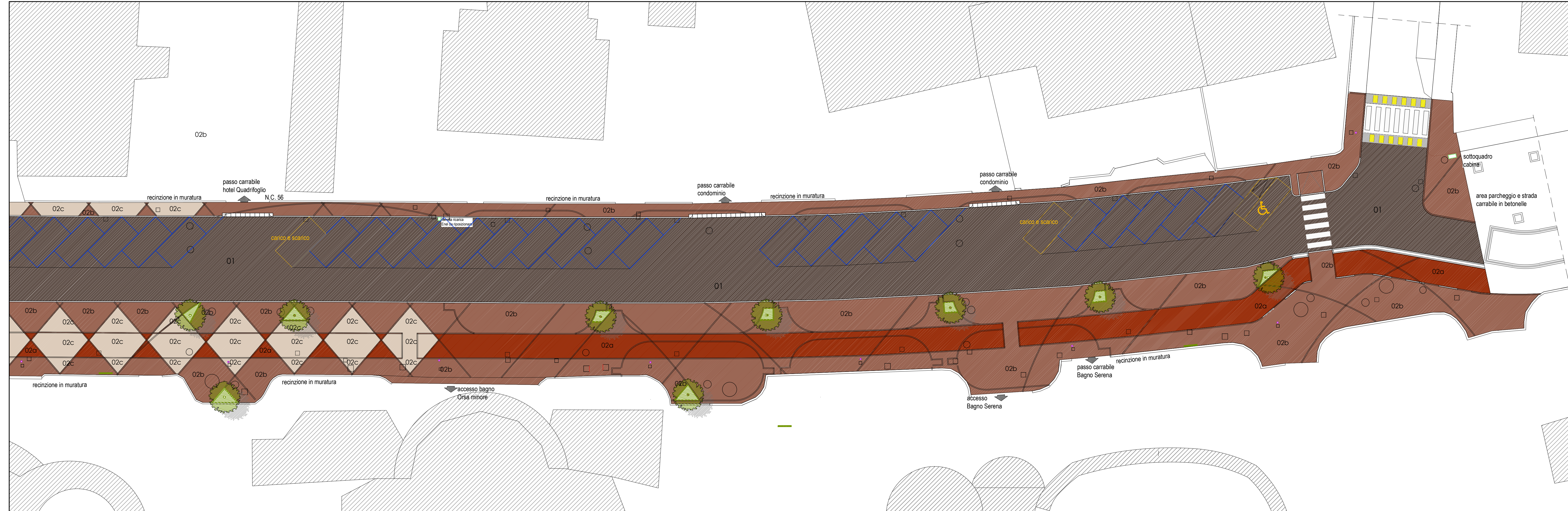
Planimetria TRATTO "B" scala 1:200
