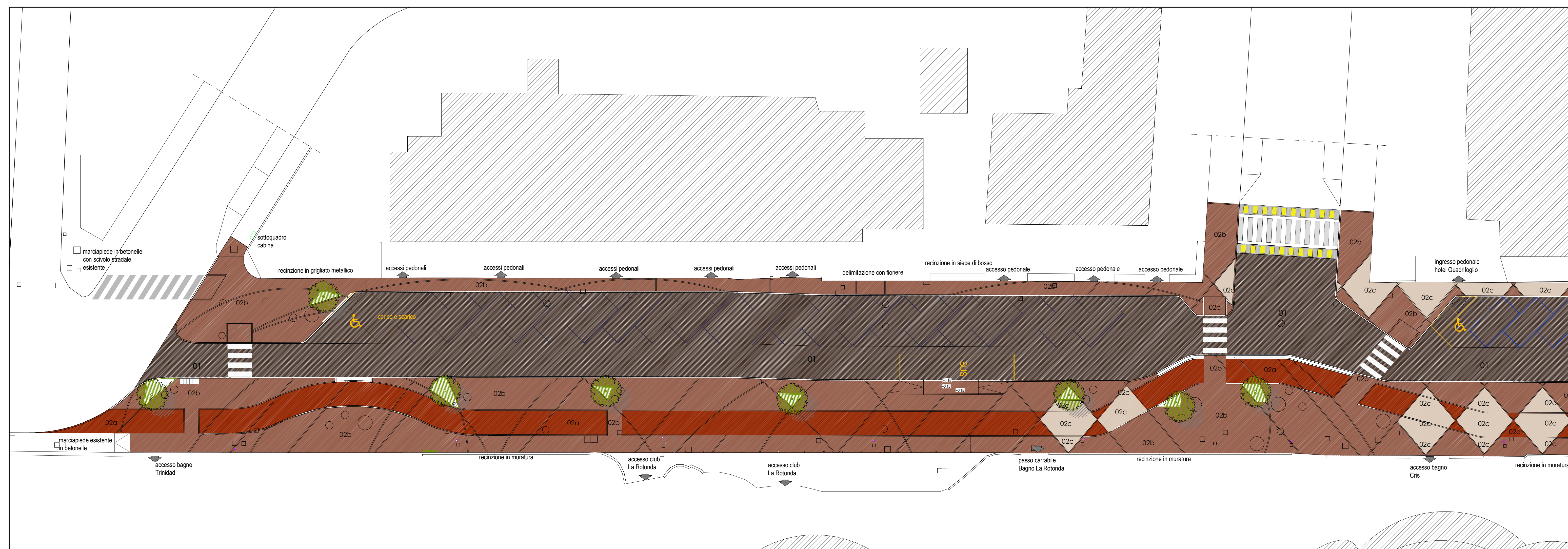
Planimetria TRATTO "A" scala 1:200
