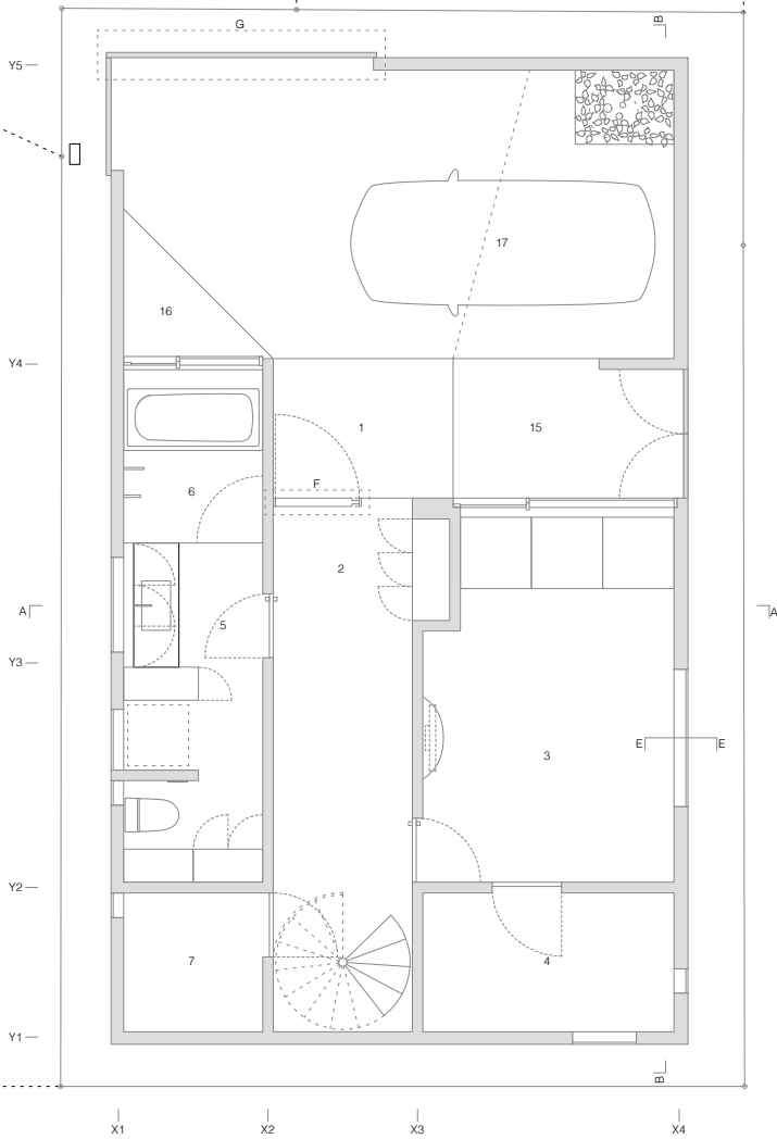
1F plan 1:100
