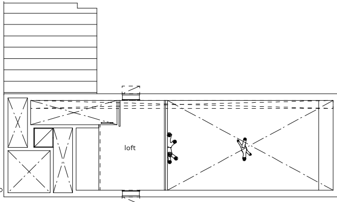
LOFT PLAN
