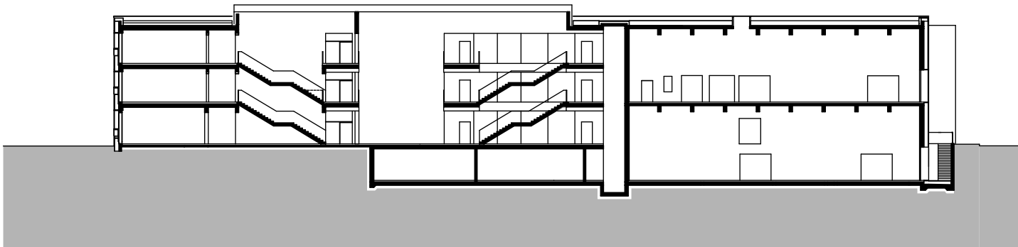
LÄNGSSCHNITT
