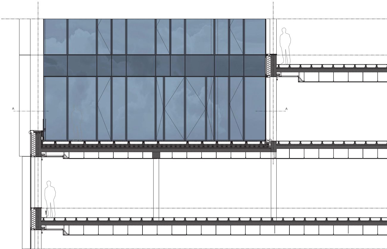
COUPE 1-1
