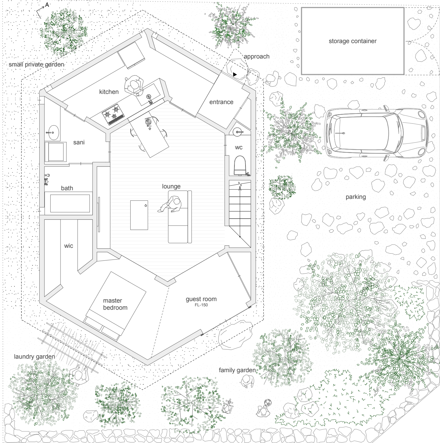
1F / SITE PLAN 1:100
