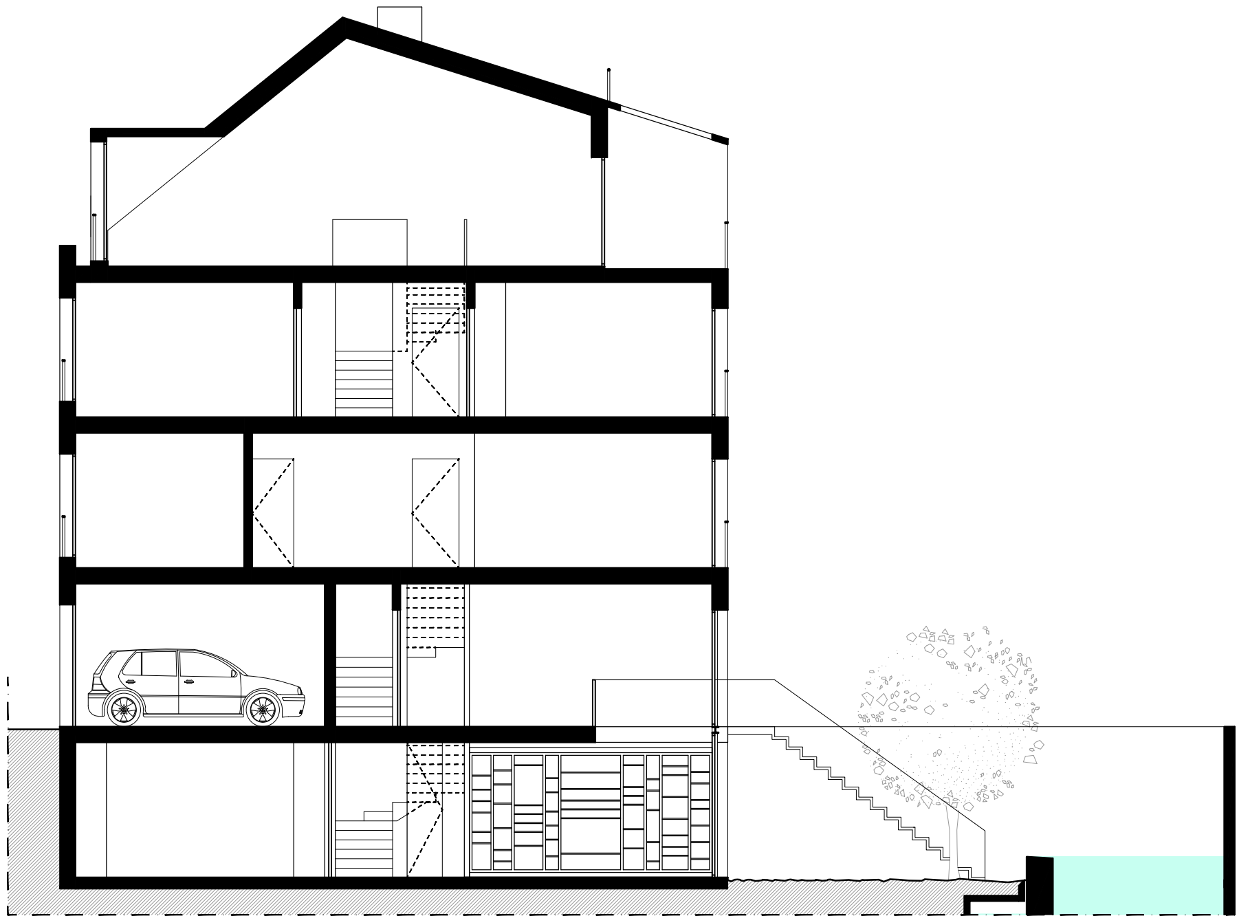
LONGITUDINAL SECTION
