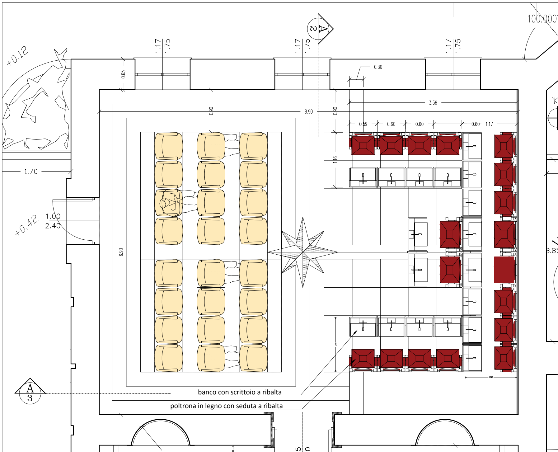
Pianta arredo sala Consiglio Comunale - Scala 1:50 -
