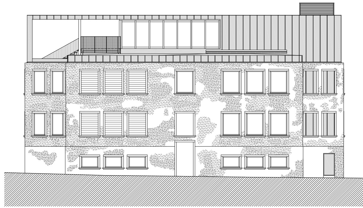
prospetto sud
