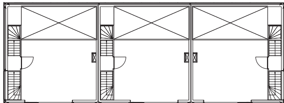
1e verdieping
