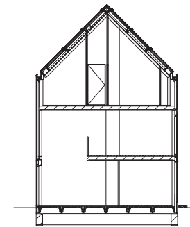
Dwarsdoorsnede
