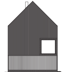
Kopgevel
