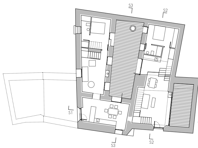
PLANTA BAJA
