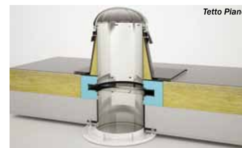
Tetto Piano
