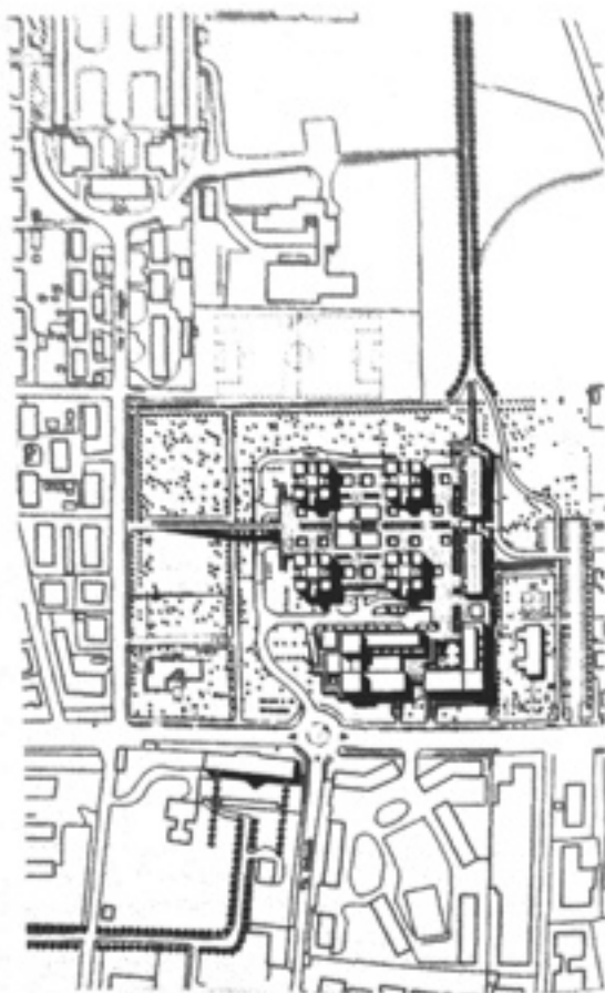
Fig. 44 Rigualificazione urbana area Ospizio a Reggio Emilia: seconda soluzione. Planimetria generale.
