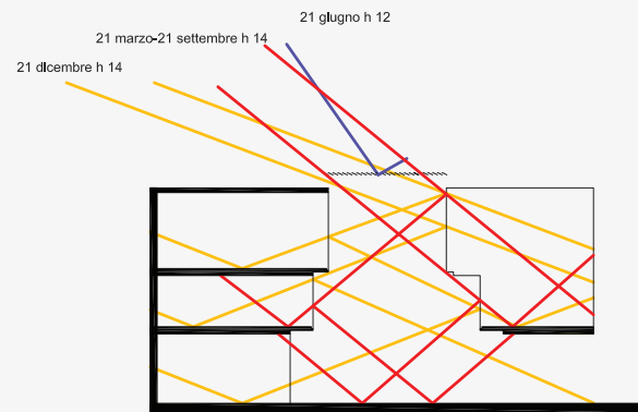
SEZIONE D
