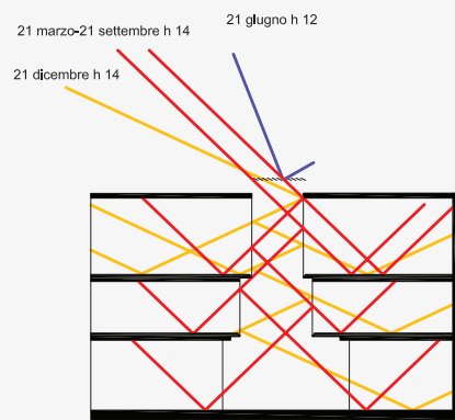
SEZIONE A
