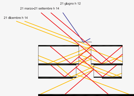
SEZIONE C
