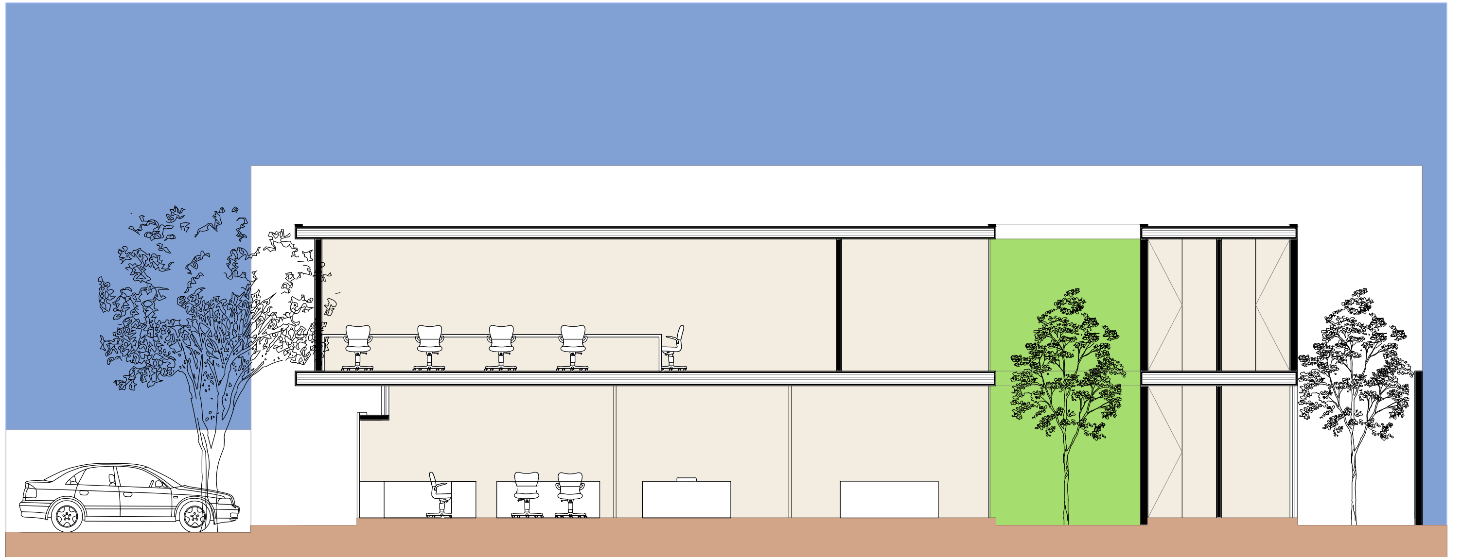
CORTE A-A'
