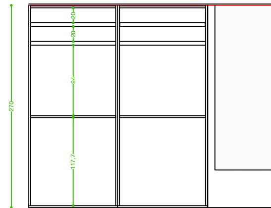
Prospetto lato porta
