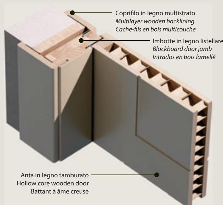
Imbotte - Plana Plana - Door jamb Intrados - Plana
