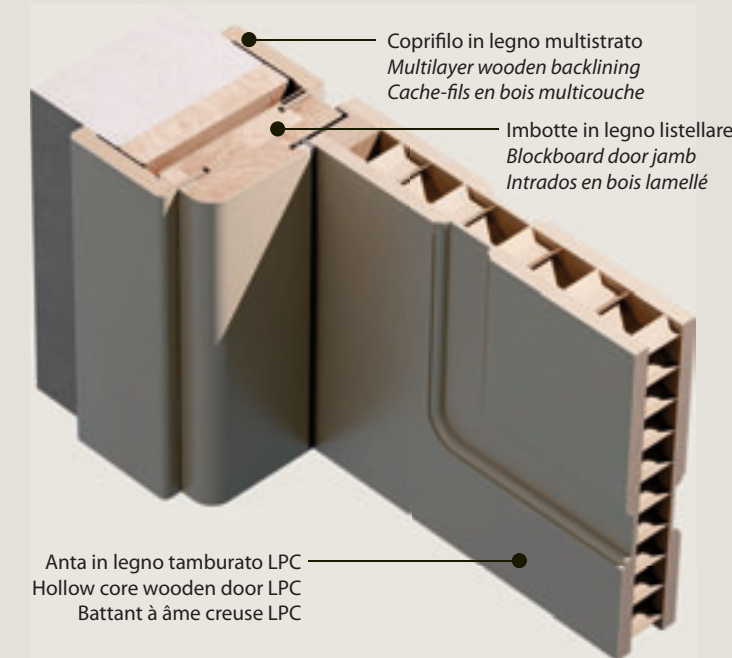
Imbotte - Raggio 10 Radius 10 - Door jamb Intrados - Rayon 10
