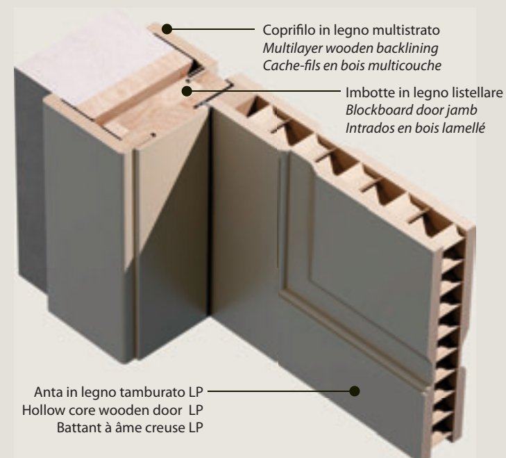
Imbotte - Plana Plana - Door jamb Intrados - Plana
