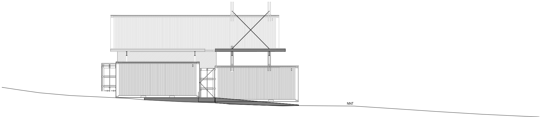
ELEVACIÓN NOR-OESTE
