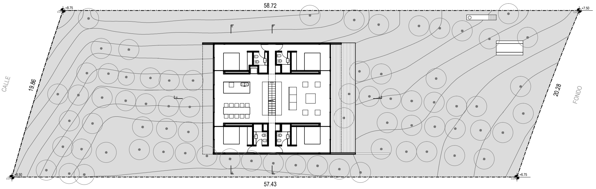
CASA L4 - PLANTA GENERAL
