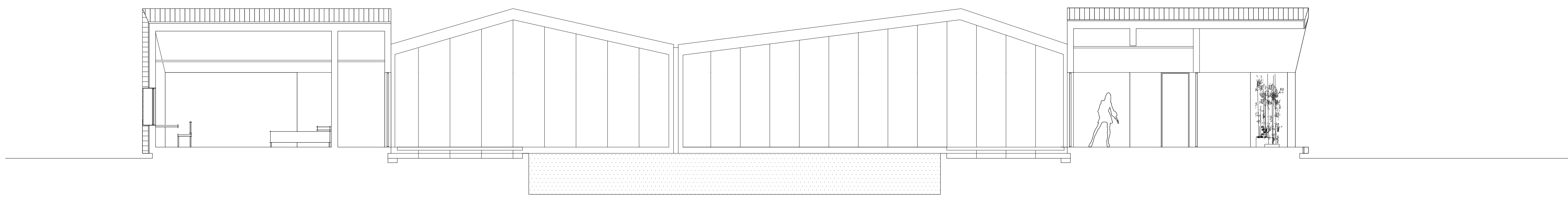
CORTE B
