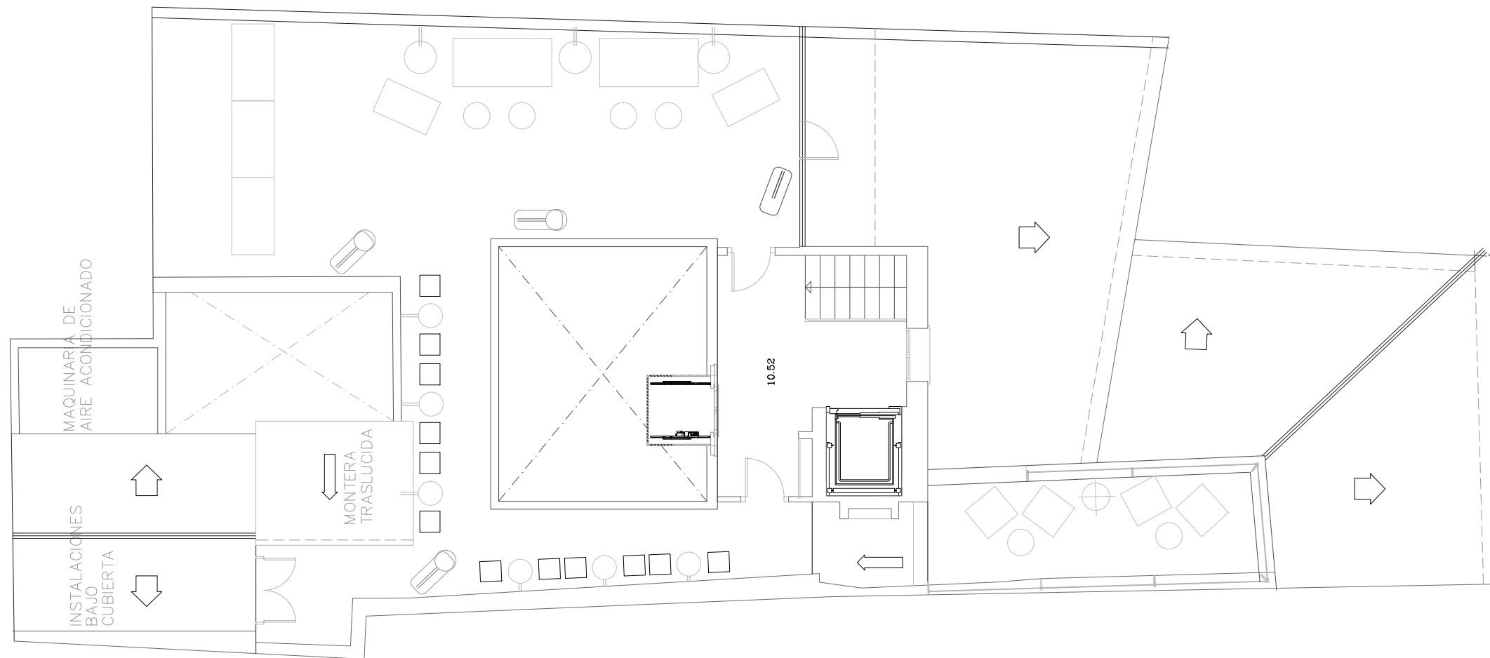
Planta - Escala 1:100
