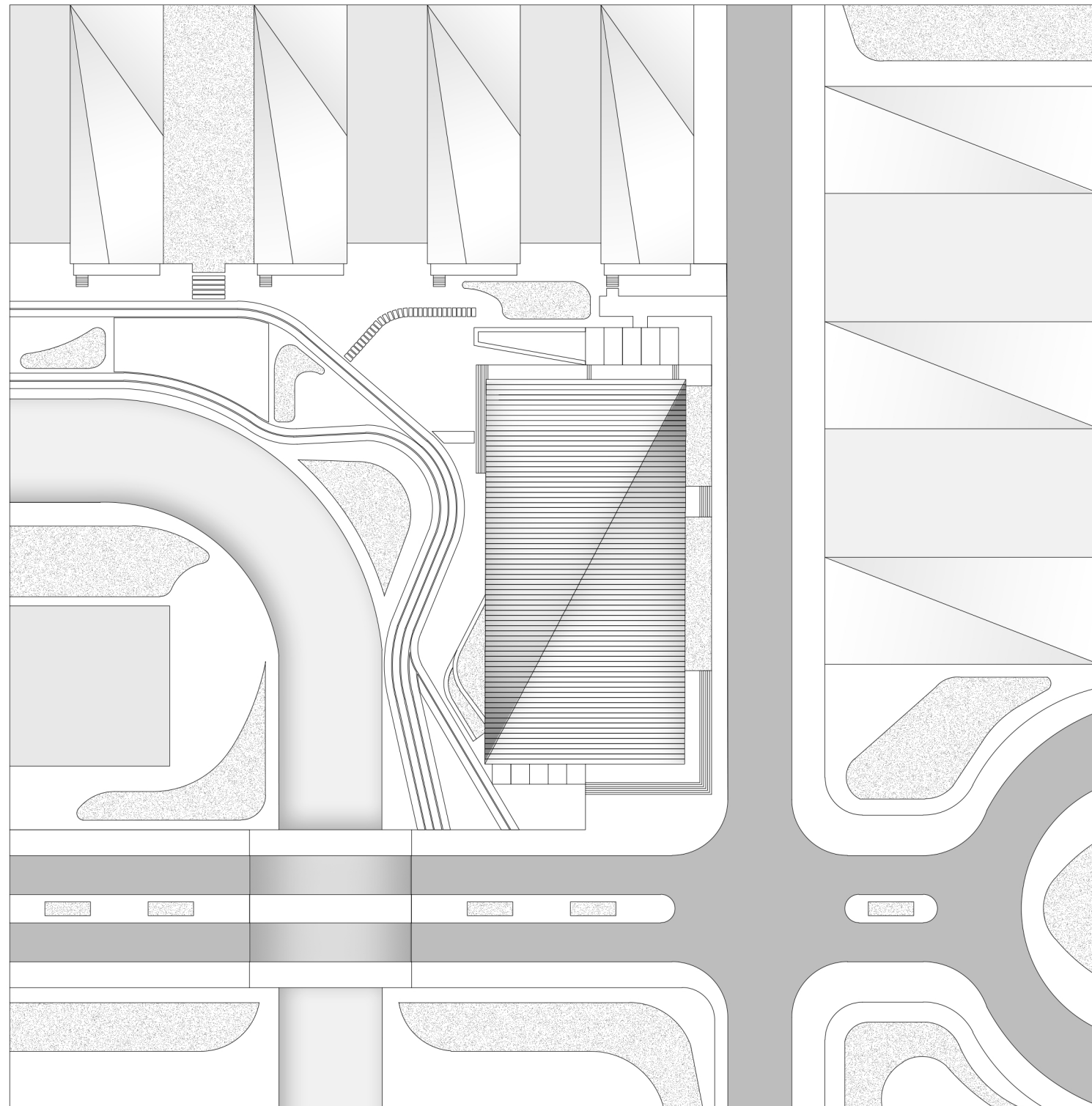
总平图 Master Plan
