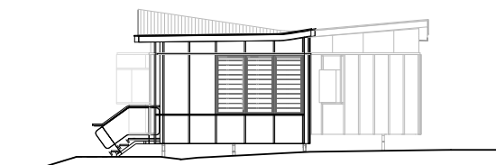
ELEVATION A
