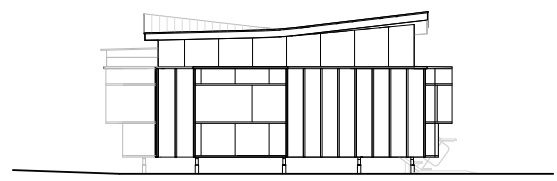
ELEVATION B
