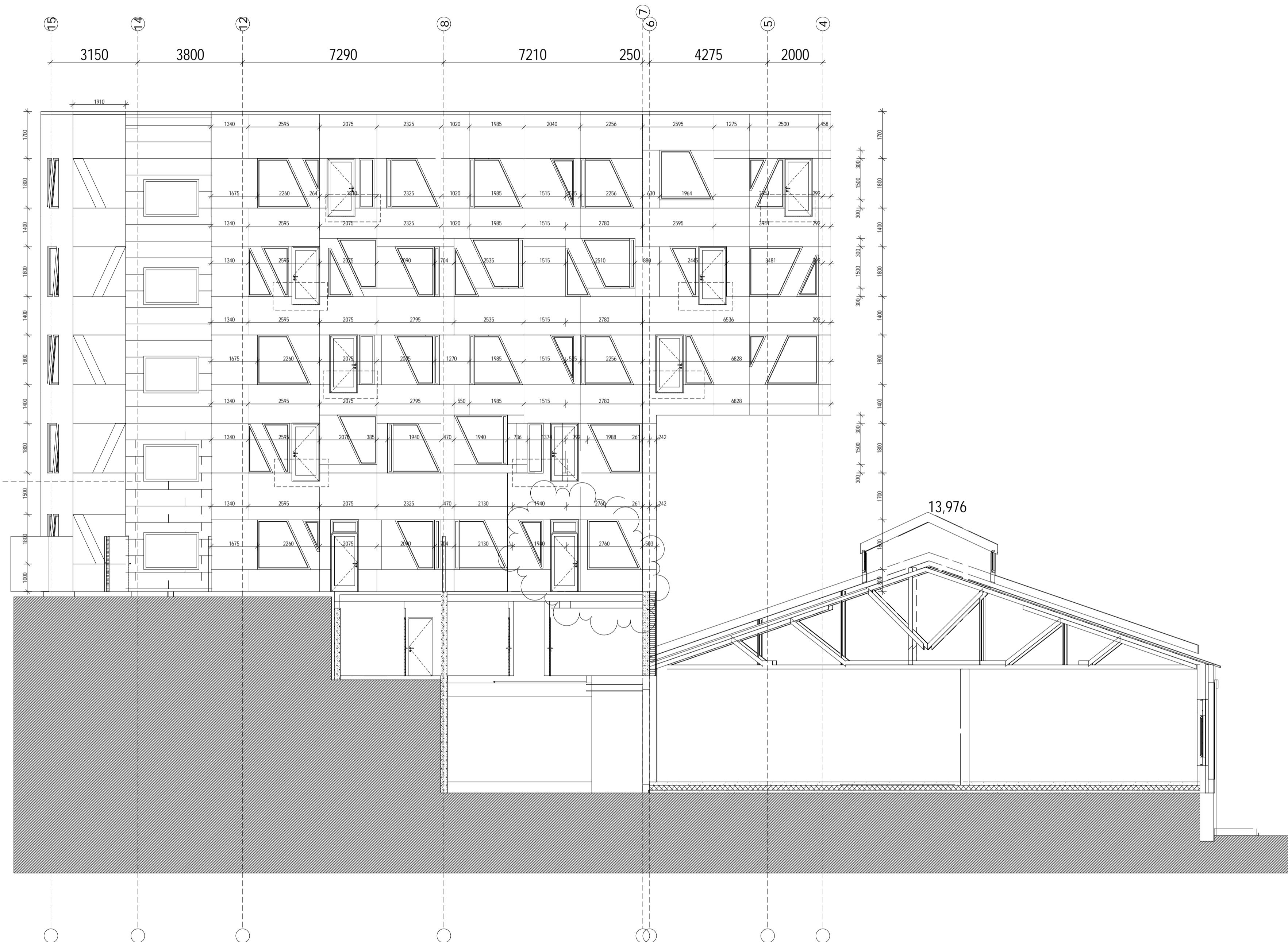
Strandlien hus D Fasade mot Verket Dato: 21.01.2014 LINK arkitektur AS
