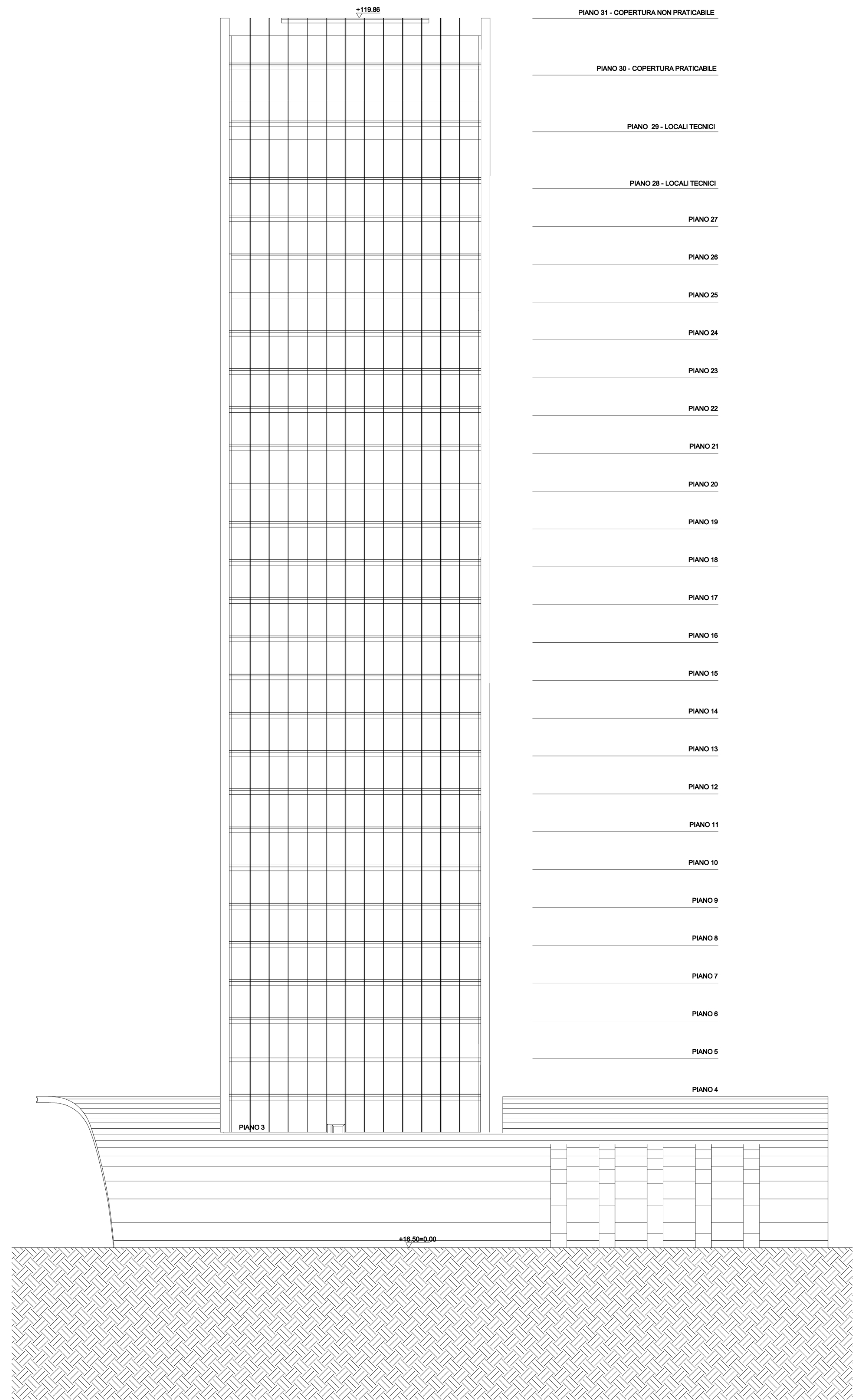
PROSPETTO B
