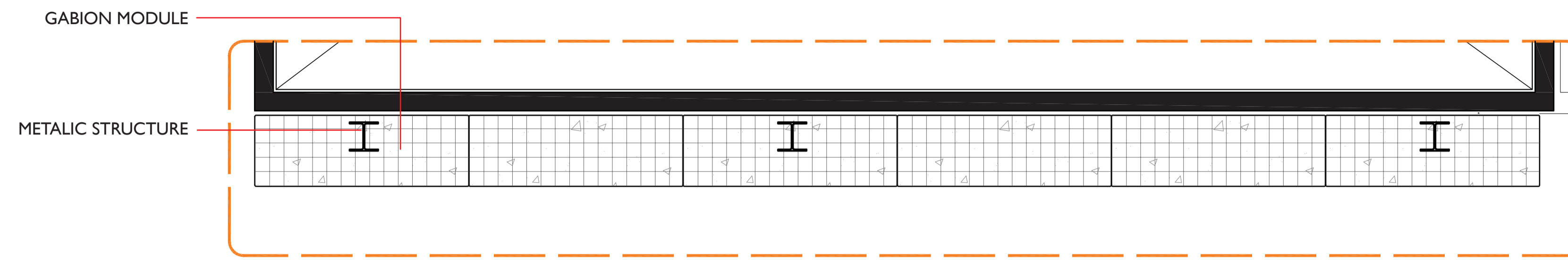
FAÇADE - PLAN 0 0.5 1 2
