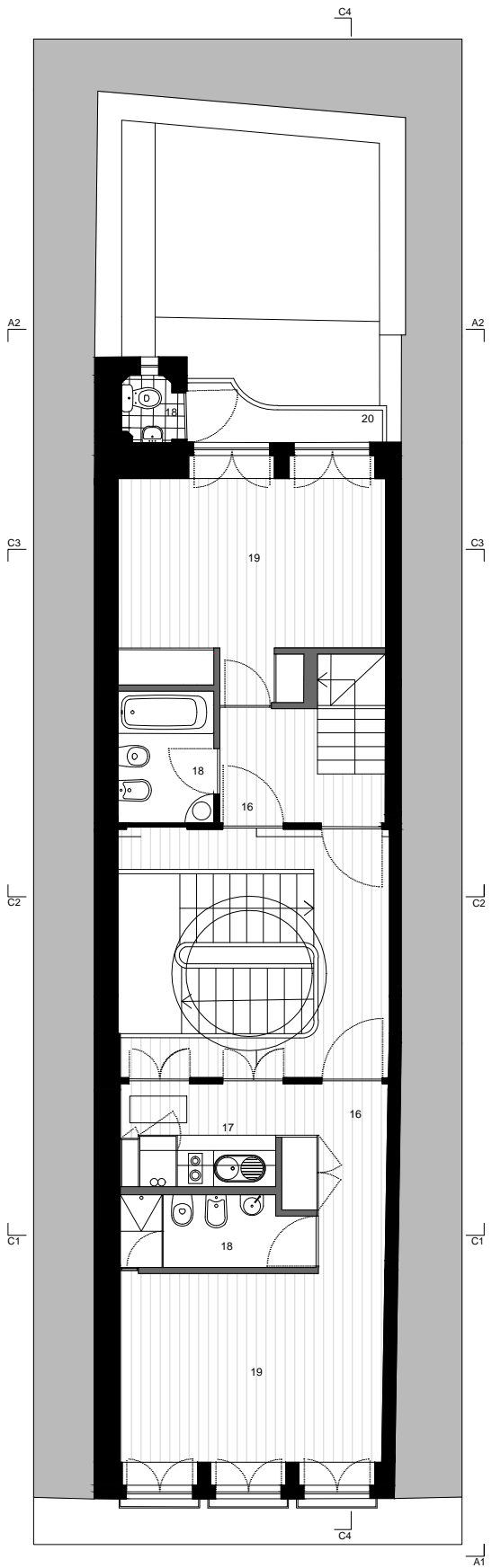
PLANTA DO PISO 2
