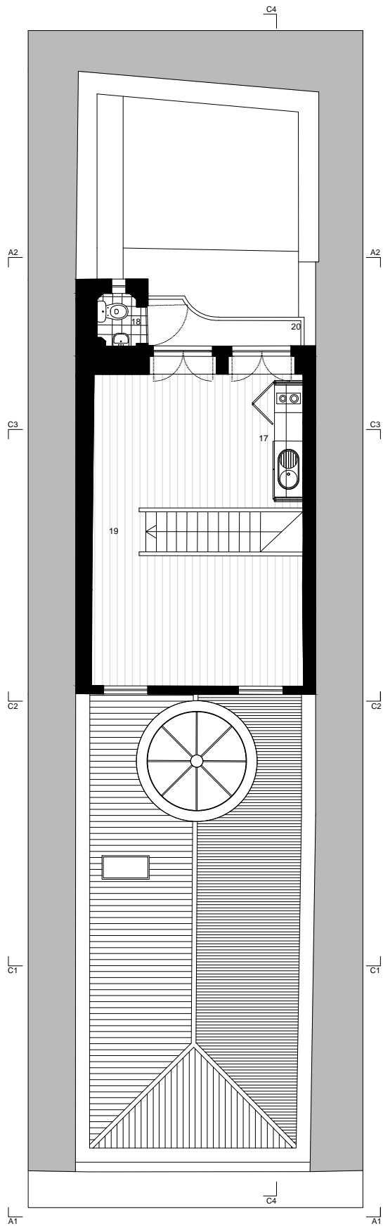
PLANTA DO PISO 3
