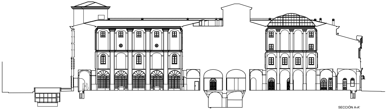
SECCIÓN A-A'
