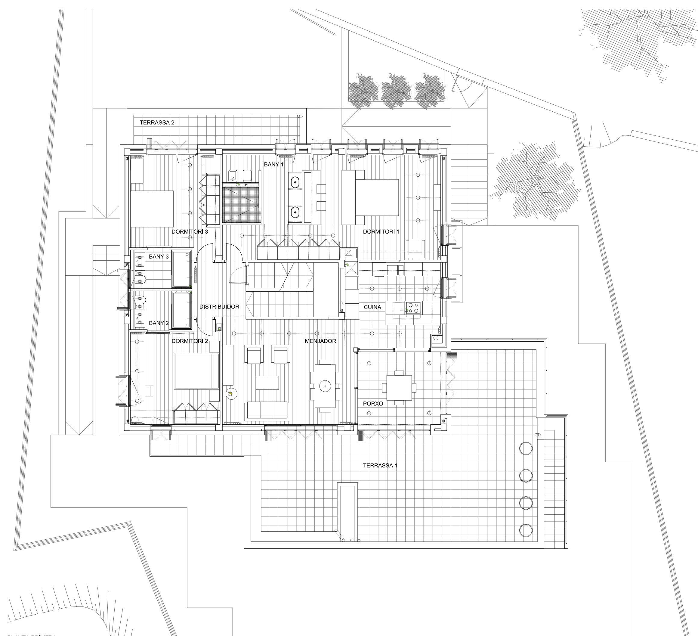
PLANTA PRIMERA
