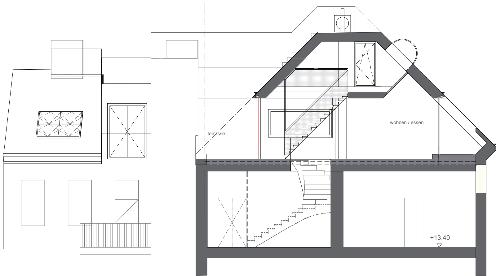
schnitt s1-s1
