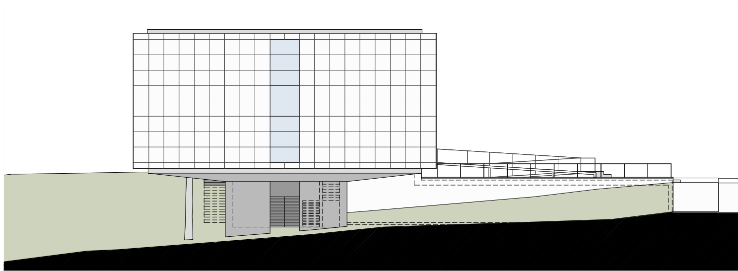
Alçado A3
