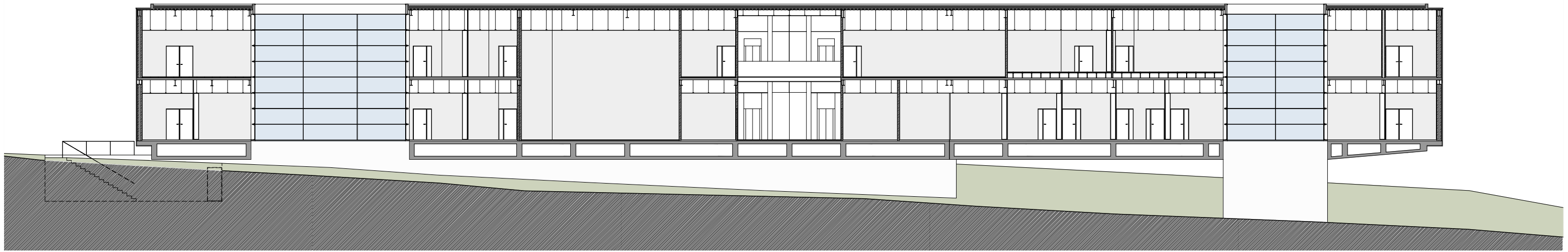
Corte C1
