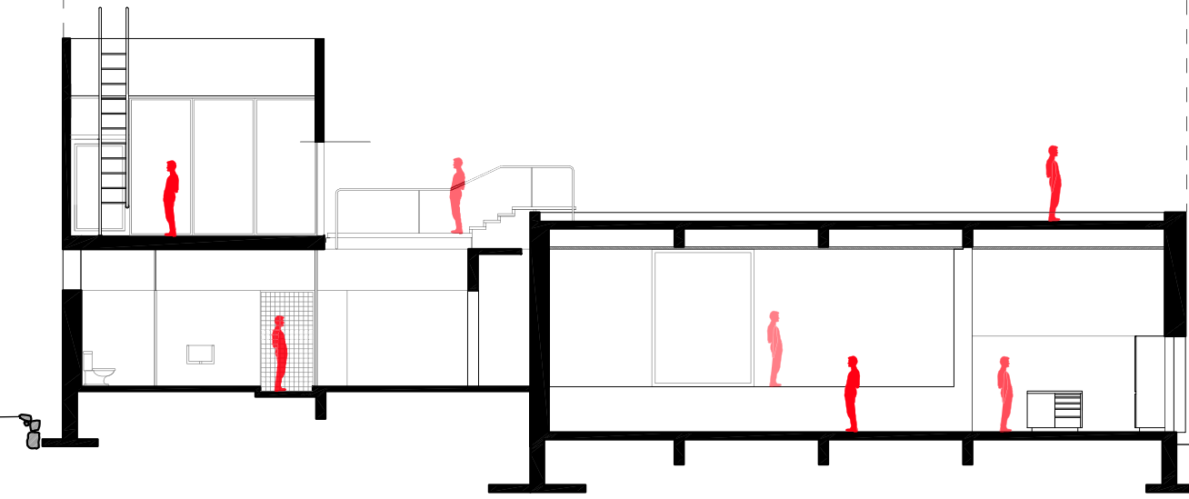
SECTION B SCALE: 1:150
