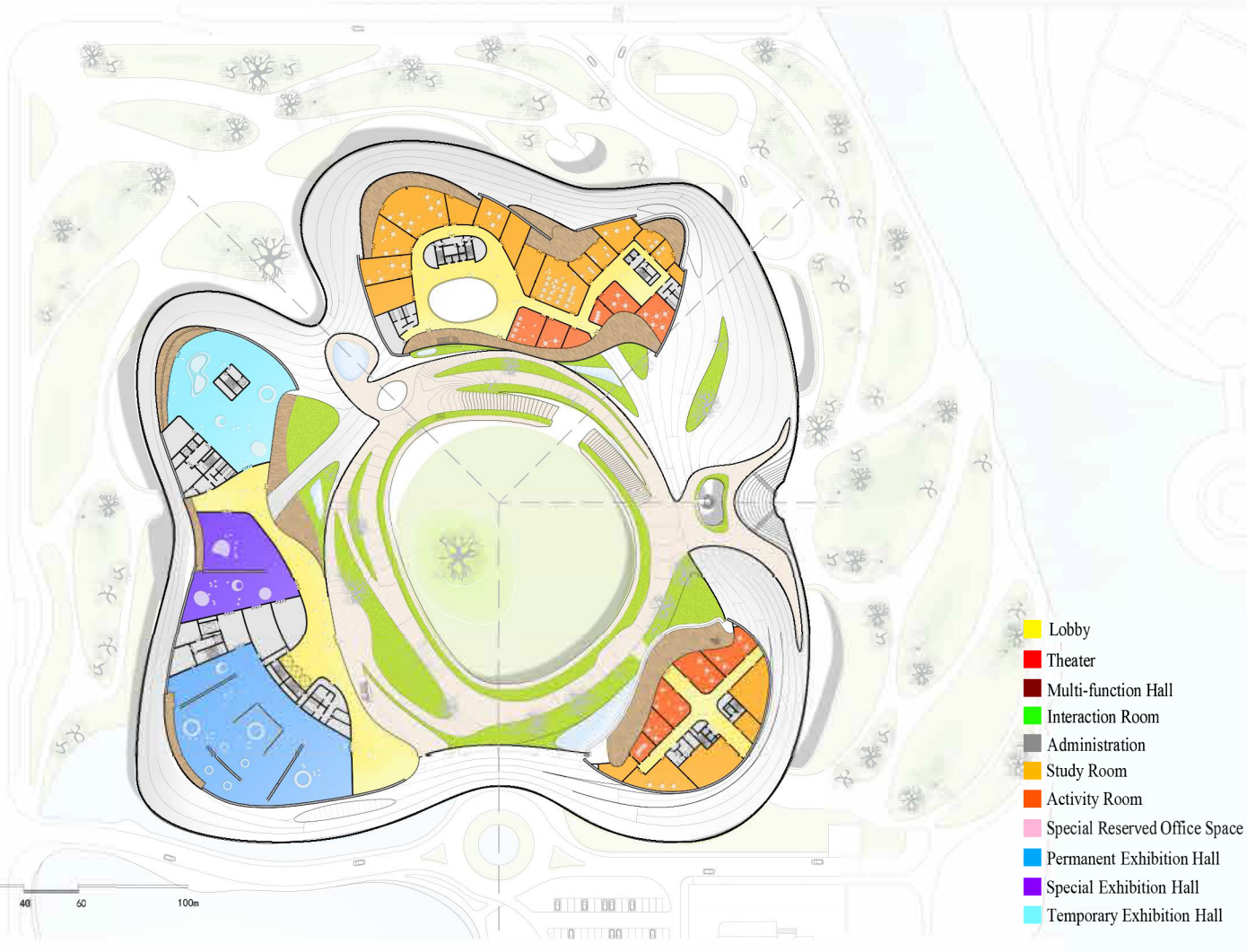
0 20 40 60 100m 二层平面 Second Floor Plan
