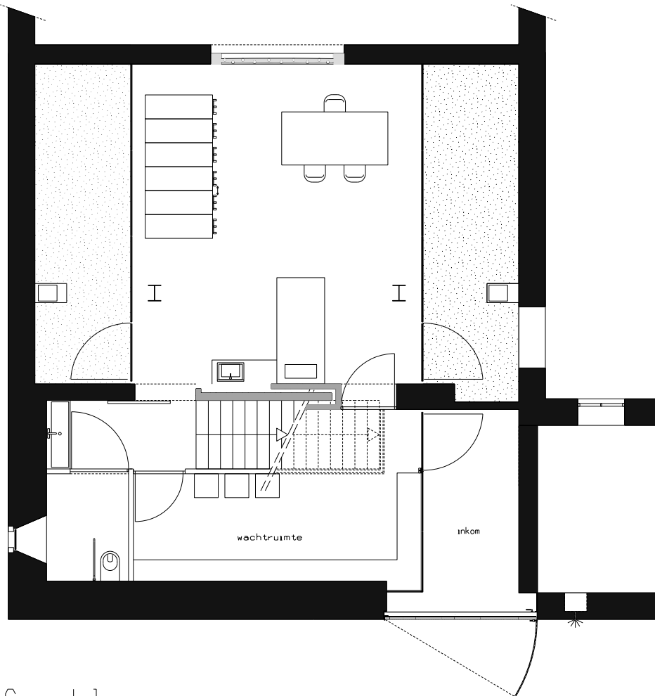
Grondplan
