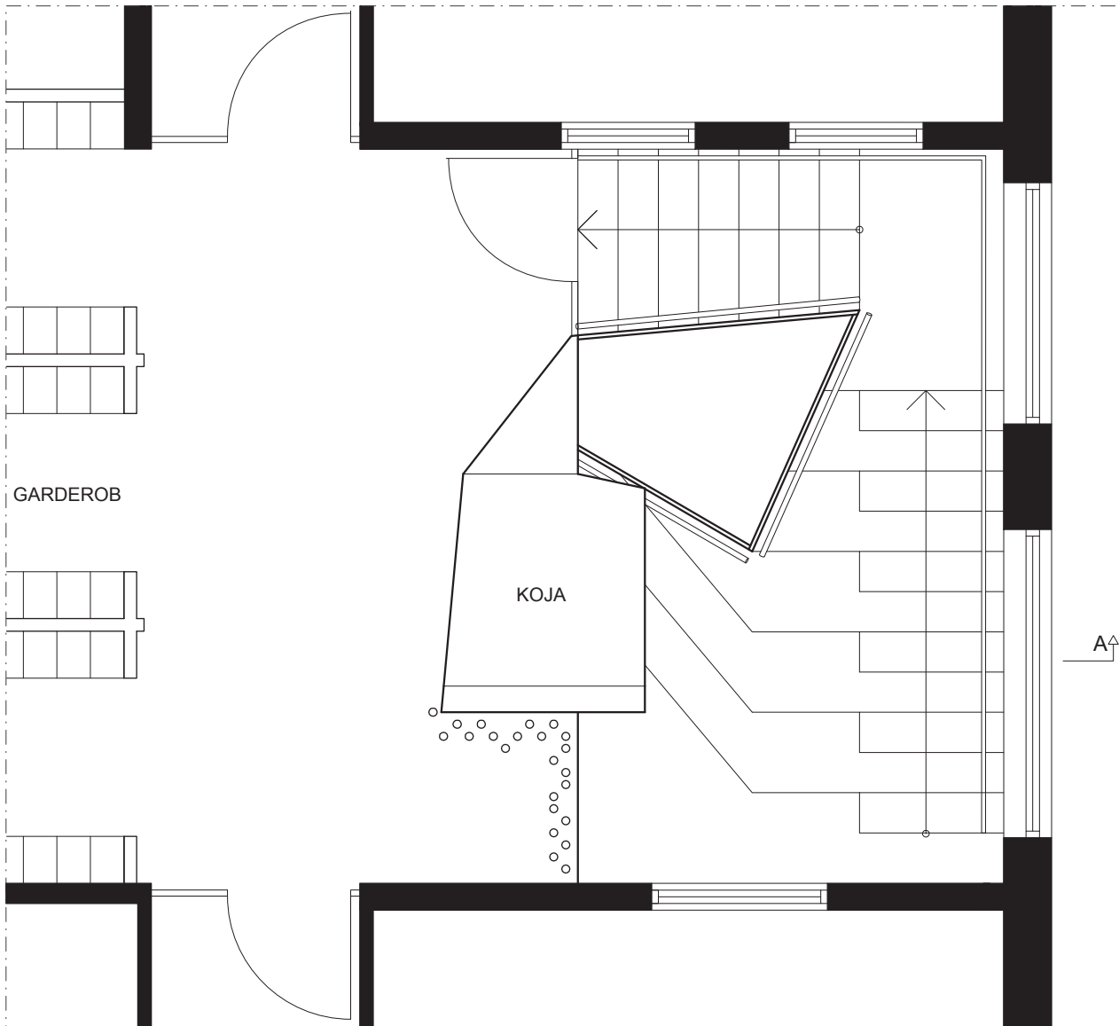
PLAN TRAPPA/KOJA 1:50
